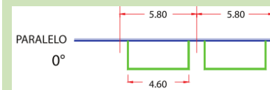
Area drenante
